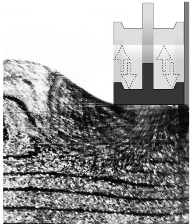
Рис. 1. Движение слоев грунта при давлении плоским штампом
